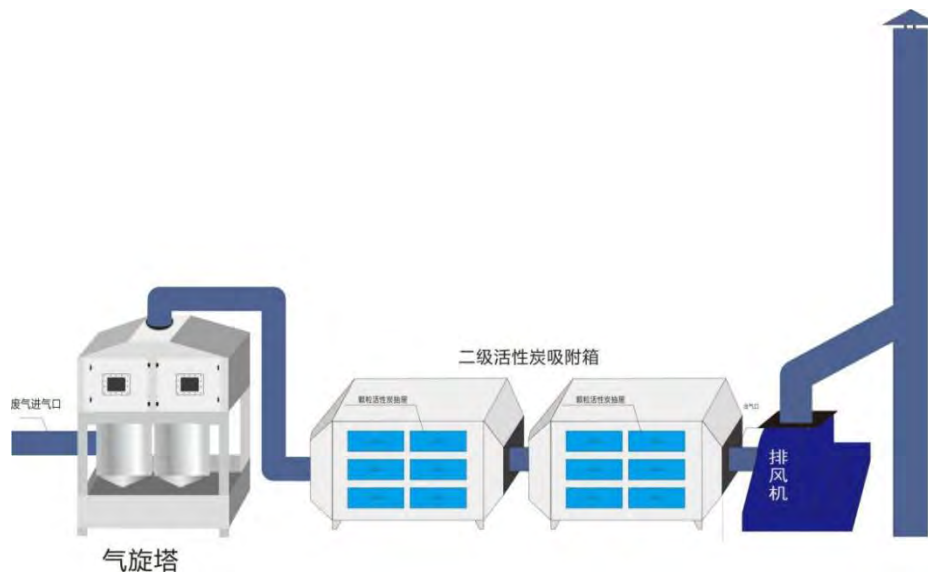
图 6 工艺流程
